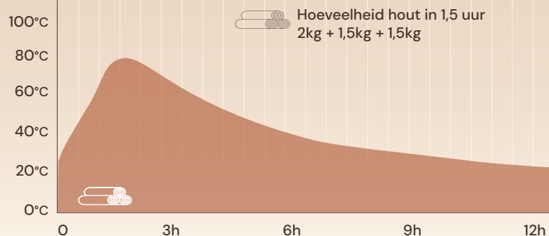
Warmte verloop van de Piccolo massakachel
